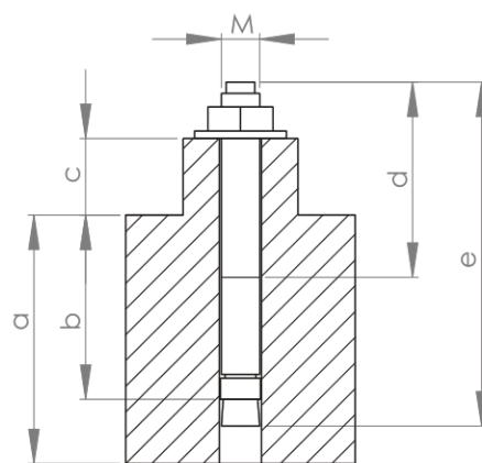
Bodendübel
