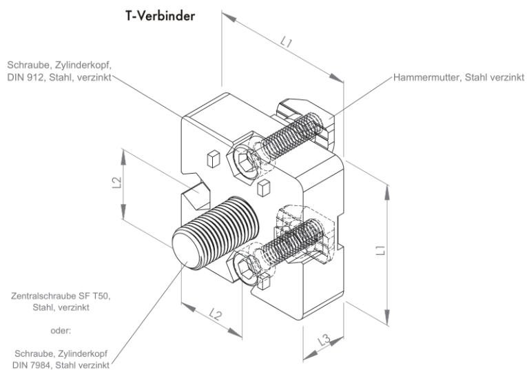
T-Verbinder
