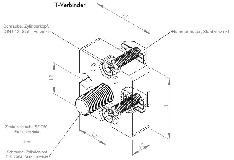
T-Verbinder
